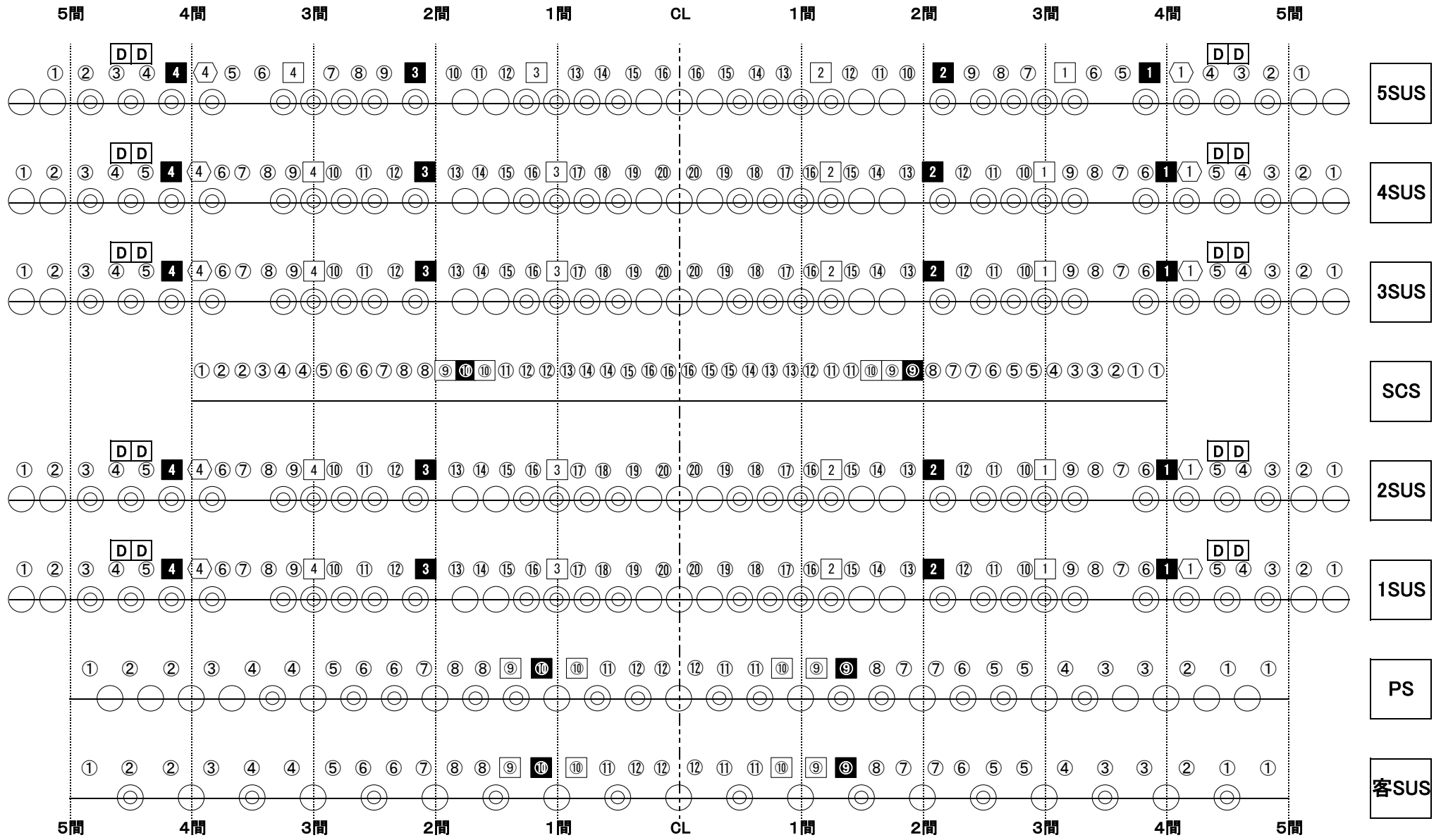
奥州市文化会館(Zホール)大ホール 基本吊り込み図
