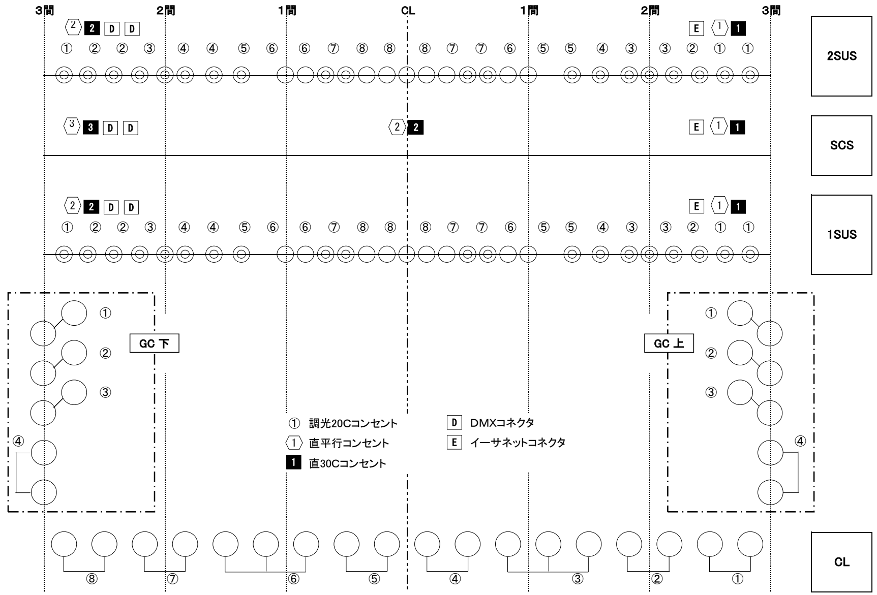
奥州市文化会館(Zホール)中ホール 基本吊り込み図
